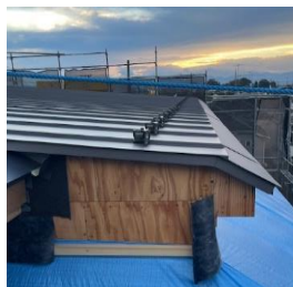
屋根板金工事(立平葺き)
