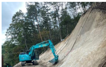
法面工事 作業風景
