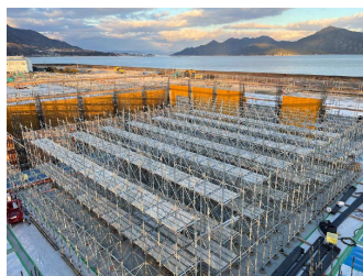
支保工足場
