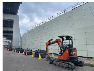
防音壁足場
